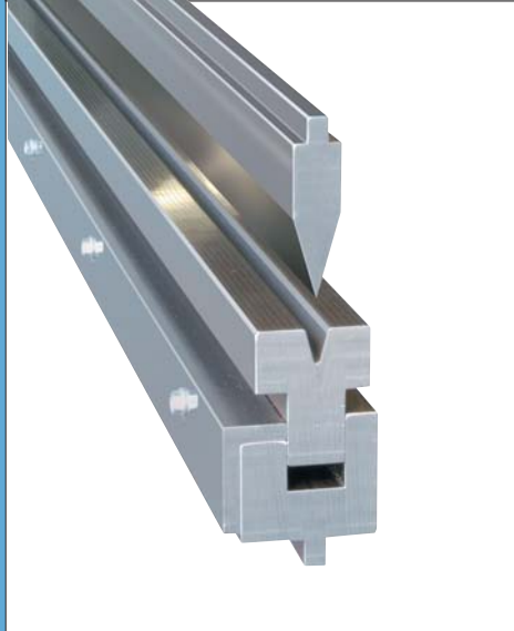
HM-3 HEMMING DIE
